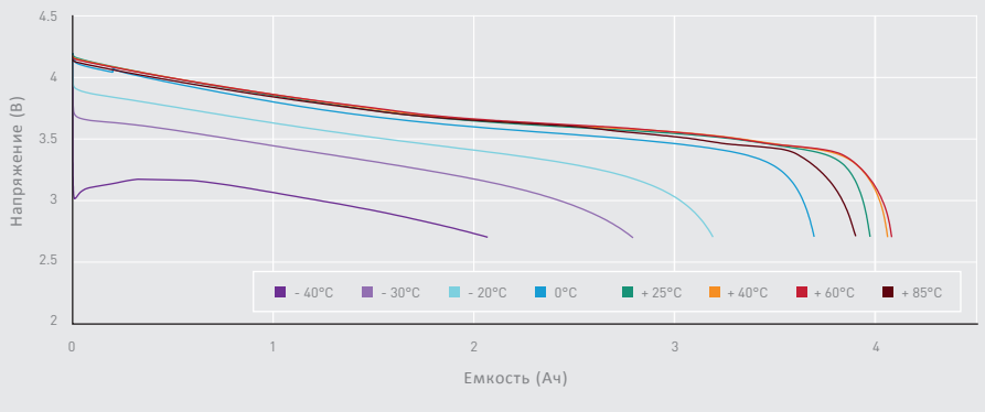
Типичные режимы разряда (0,8 А - ток C/5)
