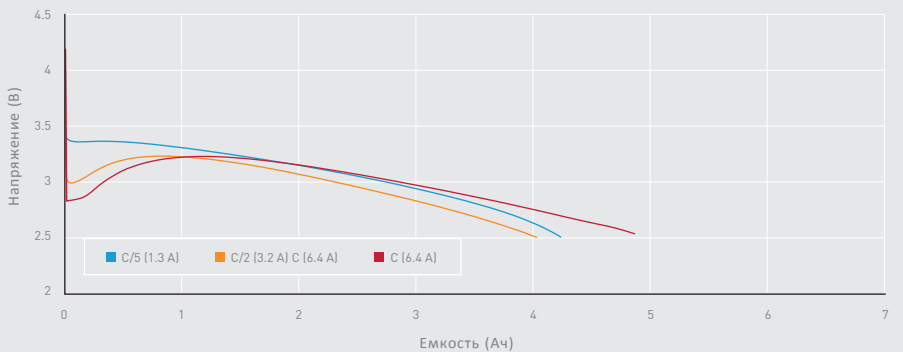
Зависимость емкости от тока при -40°C
