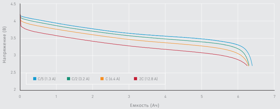
Зависимость емкости от тока при +20°C
