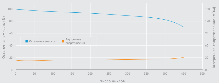
Срок службы при 20°C (заряд до 4,2 В и 3,2 А, разряд 3,0 В и 3,2 А)
